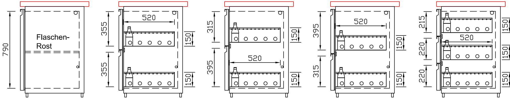
CNS-Flaschenrost mit Stellschienen Best.-Nr.: 3500 EZ-35/35 Doppelauszug 1/2-1/2 Best.-Nr.: 30210 EZ-31/39 Doppelauszug 1/3-2/3 Best.-Nr.: 30110 EZ-39/31 Doppelauszug 2/3-1/3 Best.-Nr.: 30120 EZ-22/22/22 Dreierauszug 3/3 Best.-Nr.: 30300
