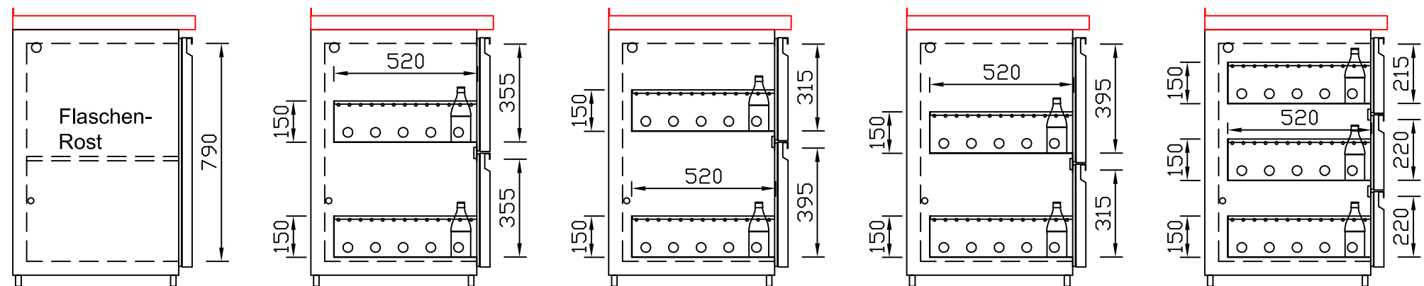
CNS-Flaschenrost mit Stellschienen Best.-Nr.: 3500
