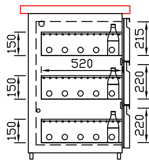
EZ-22/22/22 Dreierauszug 3/3 Best.-Nr.: 30300
