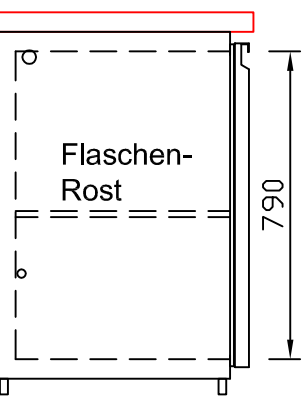
CNS-Flaschenrost mit Stellschienen Best.-Nr.: 3500
