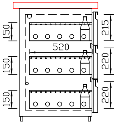
EZ-22/22/22 Dreierauszug 3/3 Best.-Nr.: 30300
