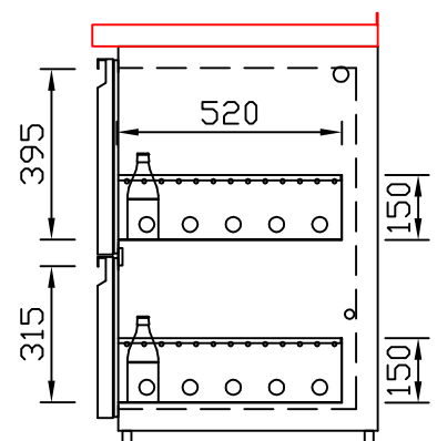
EZ-39/31 Doppelauszug 2/3-1/3 Best.-Nr.: 30120
