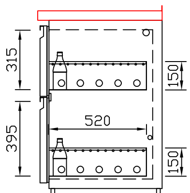
EZ-31/39 Doppelauszug 1/3-2/3 Best.-Nr.: 30110
