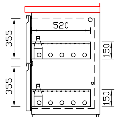
EZ-35/35 Doppelauszug 1/2-1/2 Best.-Nr.: 30210
