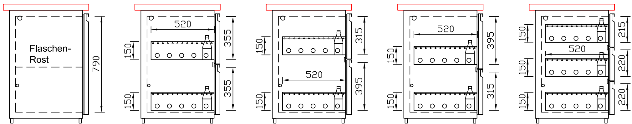
CNS-Flaschenrost mit Stellschienen Best.-Nr.: 3500 EZ-35/35 Doppelauszug 1/2-1/2 Best.-Nr.: 30210 EZ-31/39 Doppelauszug 1/3-2/3 Best.-Nr.: 30110 EZ-39/31 Doppelauszug 2/3-1/3 Best.-Nr.: 30120 EZ-22/22/22 Dreierauszug 3/3 Best.-Nr.: 30300
