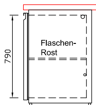
CNS-Flaschenrost mit Stellschienen Best.-Nr.: 3500
