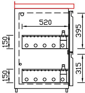
EZ-39/31 Doppelauszug 2/3-1/3 Best.-Nr.: 30120
