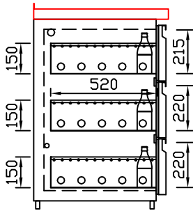
EZ-22/22/22 Dreierauszug 3/3 Best.-Nr.: 30300
