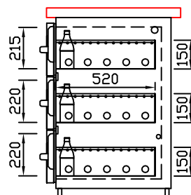
GZ-22/22/22 Dreierauszug 3/3 Best.-Nr.: 40300
