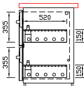
GZ-35/35 Doppelauszug 1/2-1/2 Best.-Nr.: 40210
