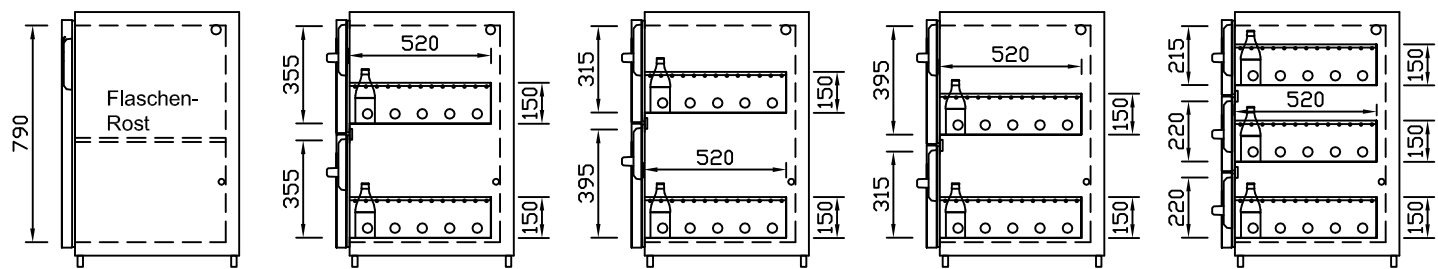
CNS-Flaschenrost mit Stellschienen Best.-Nr.: 3500
