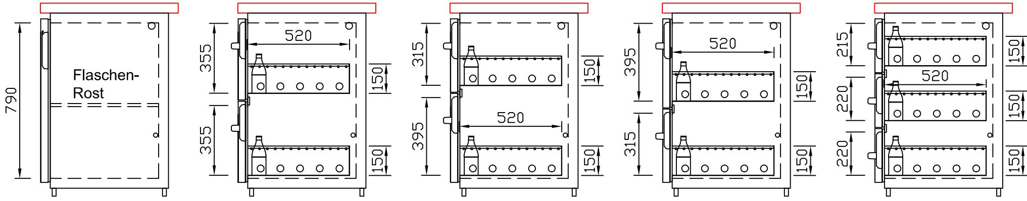
CNS-Flaschenrost mit Stellschienen Best.-Nr.: 3500 GZ-35/35 Doppelauszug 1/2-1/2 Best.-Nr.: 40210 GZ-31/39 Doppelauszug 1/3-2/3 Best.-Nr.: 40110 GZ-39/31 Doppelauszug 2/3-1/3 Best.-Nr.: 40120 GZ-22/22/22 Dreierauszug 3/3 Best.-Nr.: 40300
