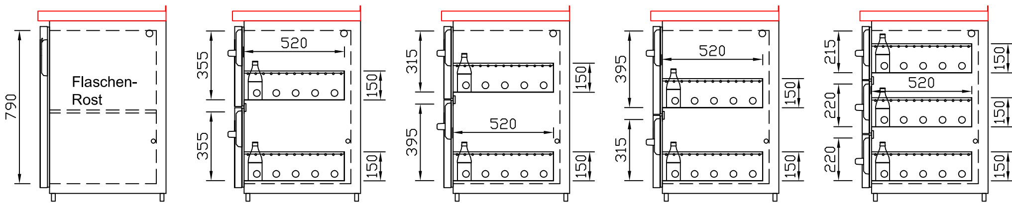
CNS-Flaschenrost mit Stellschienen Best.-Nr.: 3500 GZ-35/35 Doppelauszug 1/2-1/2 Best.-Nr.: 40210 GZ-31/39 Doppelauszug 1/3-2/3 Best.-Nr.: 40110 GZ-39/31 Doppelauszug 2/3-1/3 Best.-Nr.: 40120 GZ-22/22/22 Dreierauszug 3/3 Best.-Nr.: 40300
