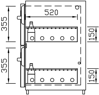
GZ-35/35 Doppelauszug 1/2-1/2 Best.-Nr.: 40210
