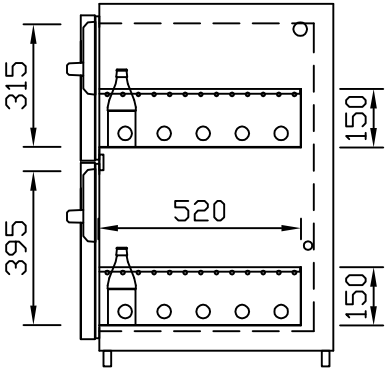
GZ-31/39 Doppelauszug 1/3-2/3 Best.-Nr.: 40110
