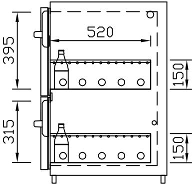
GZ-39/31 Doppelauszug 2/3-1/3 Best.-Nr.: 40120
