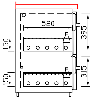
GZ-39/31 Doppelauszug 2/3-1/3 Best.-Nr.: 40120
