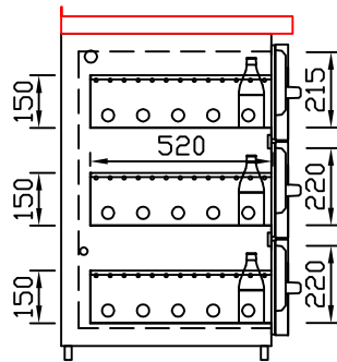
GZ-22/22/22 Dreierauszug 3/3 Best.-Nr.: 40300
