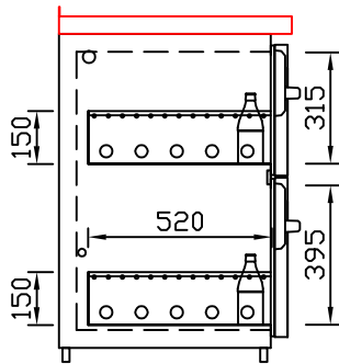
GZ-31/39 Doppelauszug 1/3-2/3 Best.-Nr.: 40110
