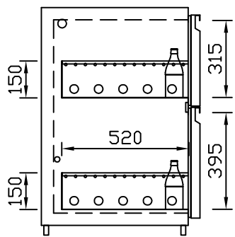
EZ-31/39 Doppelauszug 1/3-2/3 Best.-Nr.: 30110
