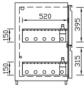
EZ-39/31 Doppelauszug 2/3-1/3 Best.-Nr.: 30120
