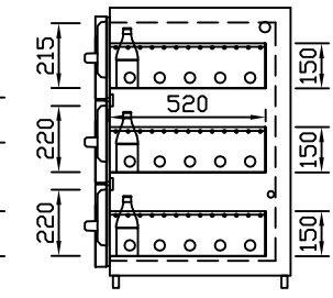
GZ-22/22/22 Dreierauszug 3/3 Best.-Nr.: 40300
