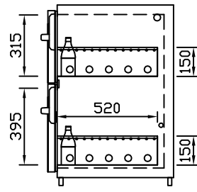
GZ-31/39 Doppelauszug 1/3-2/3 Best.-Nr.: 40110
