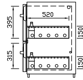
GZ-39/31 Doppelauszug 2/3-1/3 Best.-Nr.: 40120
