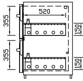
GZ-35/35 Doppelauszug 1/2-1/2 Best.-Nr.: 40210
