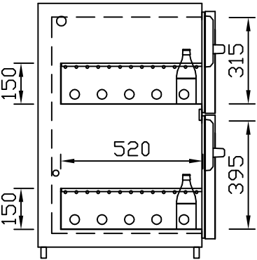
GZ-31/39 Doppelauszug 1/3-2/3 Best.-Nr.: 40110
