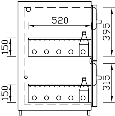
GZ-39/31 Doppelauszug 2/3-1/3 Best.-Nr.: 40120
