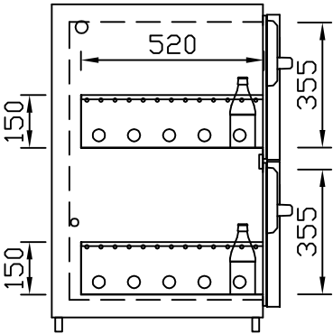
GZ-35/35 Doppelauszug 1/2-1/2 Best.-Nr.: 40210
