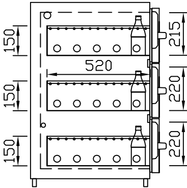
GZ-22/22/22 Dreierauszug 3/3 Best.-Nr.: 40300
