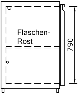
CNS-Flaschenrost mit Stellschienen Best.-Nr.: 3500
