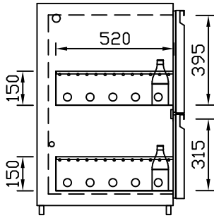
EZ-39/31 Doppelauszug 2/3-1/3 Best.-Nr.: 30120
