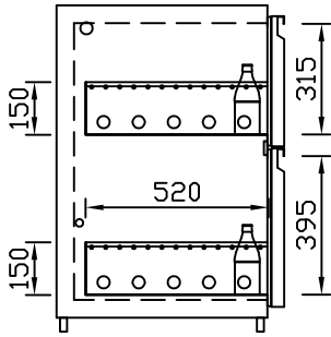
EZ-31/39 Doppelauszug 1/3-2/3 Best.-Nr.: 30110
