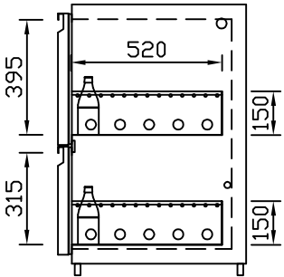
EZ-39/31 Doppelauszug 2/3-1/3 Best.-Nr.: 30120
