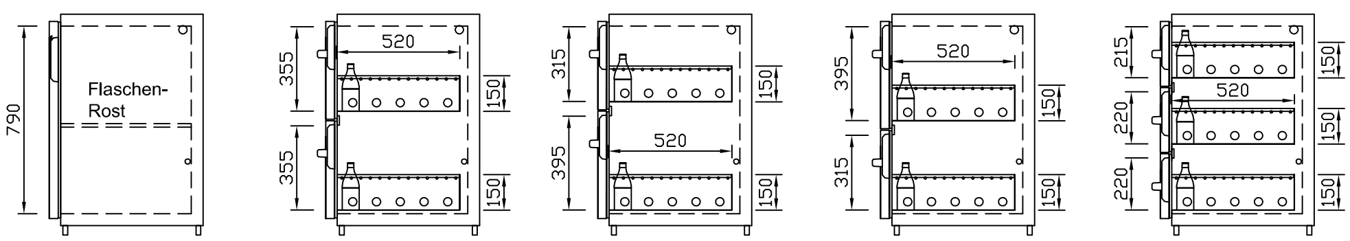
CNS-Flaschenrost mit Stellschienen Best.-Nr.: 3500 GZ-35/35 Doppelauszug 1/2-1/2 Best.-Nr.: 40210 GZ-31/39 Doppelauszug 1/3-2/3 Best.-Nr.: 40110 GZ-39/31 Doppelauszug 2/3-1/3 Best.-Nr.: 40120 GZ-22/22/22 Dreierauszug 3/3 Best.-Nr.: 40300
