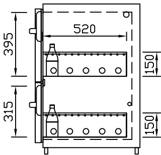
GZ-39/31 Doppelauszug 2/3-1/3 Best.-Nr.: 40120
