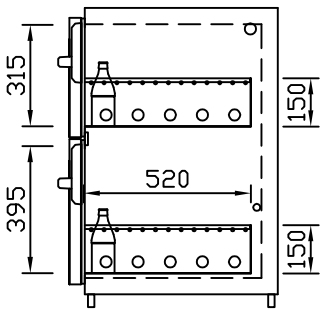
GZ-31/39 Doppelauszug 1/3-2/3 Best.-Nr.: 40110
