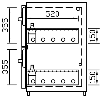
GZ-35/35 Doppelauszug 1/2-1/2 Best.-Nr.: 40210
