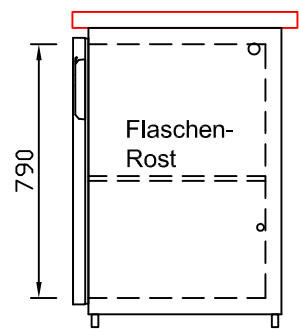
CNS-Flaschenrost mit Stellschienen Best.-Nr.: 3500
