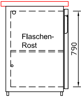
CNS-Flaschenrost mit Stellschienen Best.-Nr.: 3500
