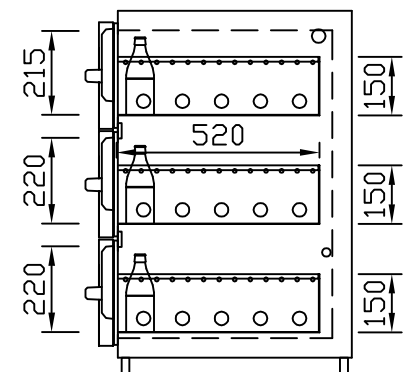
GZ-22/22/22 Dreierauszug 3/3 Best.-Nr.: 40300
