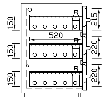
GZ-22/22/22 Dreierauszug 3/3 Best.-Nr.: 40300
