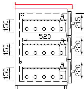
GZ-22/22/22 Dreierauszug 3/3 Best.-Nr.: 40300
