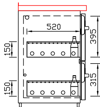
GZ-39/31 Doppelauszug 2/3-1/3 Best.-Nr.: 40120
