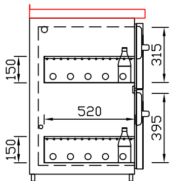
GZ-31/39 Doppelauszug 1/3-2/3 Best.-Nr.: 40110
