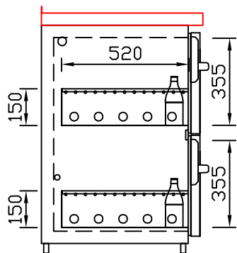
GZ-35/35 Doppelauszug 1/2-1/2 Best.-Nr.: 40210
