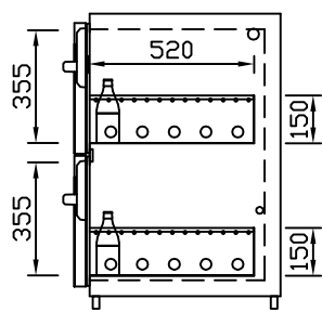
GZ-35/35 Doppelauszug 1/2-1/2 Best.-Nr.: 40210
