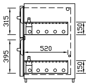
GZ-31/39 Doppelauszug 1/3-2/3 Best.-Nr.: 40110
