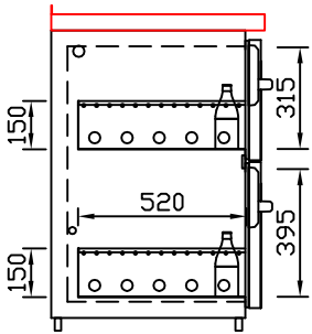
GZ-31/39 Doppelauszug 1/3-2/3 Best.-Nr.: 40110
