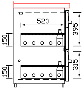
GZ-39/31 Doppelauszug 2/3-1/3 Best.-Nr.: 40120
