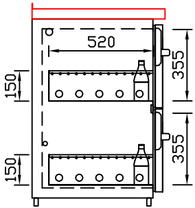
GZ-35/35 Doppelauszug 1/2-1/2 Best.-Nr.: 40210
