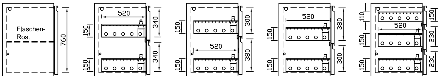
CNS-Flaschenrost mit Stellschienen Best.-Nr.: 3500
