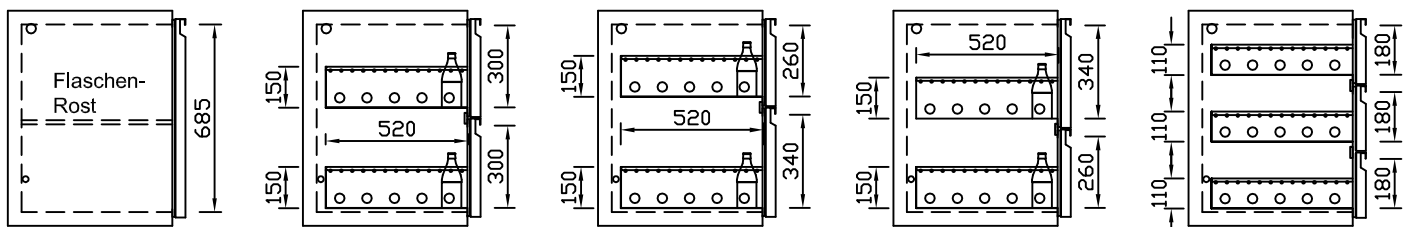
CNS-Flaschenrost mit Stellschienen Best.-Nr.: 3500
