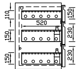
EZ-15/23/23 Dreierauszug 3/3 Best.-Nr.: 30300-860
