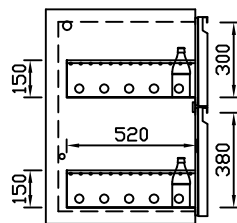
EZ-30/38 Doppelauszug 1/3-2/3 Best.-Nr.: 30110-860
