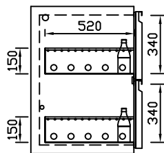
EZ-34/34 Doppelauszug 1/2-1/2 Best.-Nr.: 30210-860
