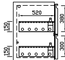
EZ-38/30 Doppelauszug 2/3-1/3 Best.-Nr.: 30120-860
