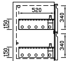
EZ-34/34 Doppelauszug 1/2-1/2 Best.-Nr.: 30210-860
