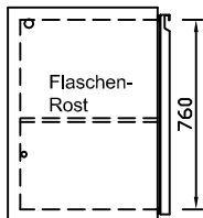
CNS-Flaschenrost mit Stellschienen Best.-Nr.: 3500
