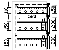
EZ-15/23/23 Dreierauszug 3/3 Best.-Nr.: 30300-860
