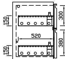
EZ-30/38 Doppelauszug 1/3-2/3 Best.-Nr.: 30110-860
